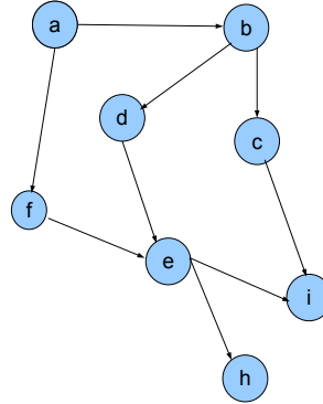
Figura 3.1: Representación de un grafo dirigido.
